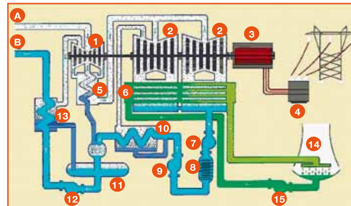
Schéma jaderné elektrárny
