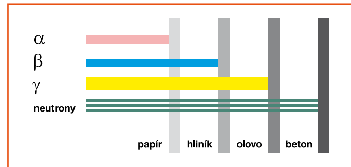
Průnik záření různými druhy materiálů
